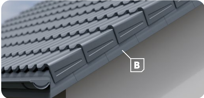
Drift 150 Długość efektywna: 350 mm Wysokość: 150 mm
